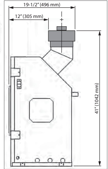
Foyer Linear, évent dessus avec raccord colinéaire
