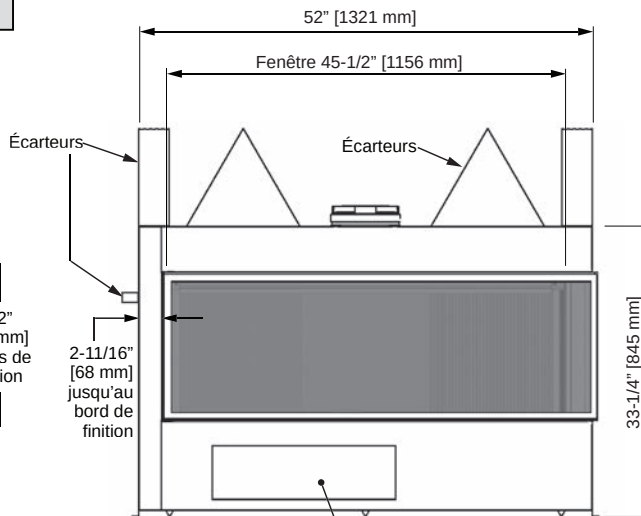
Vu du devant (foyer R montré)
