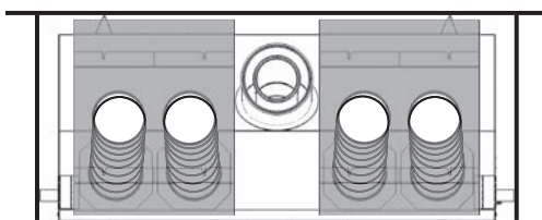
Sorties sur dessus (cantonnière) avec DK7 Note : Lorsque le LDK7 est utilisé, la sortie d'air chaud doit être dans la même pièce que le foyer.
