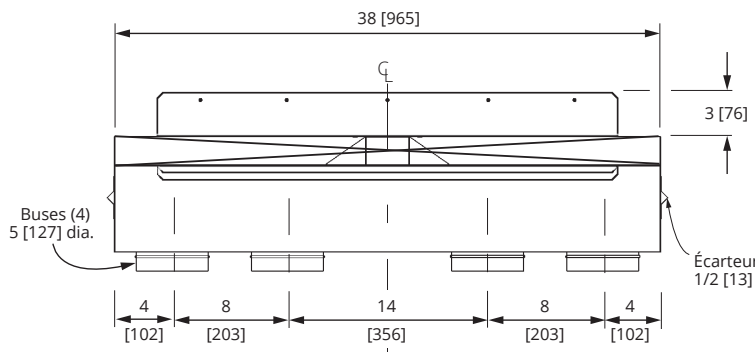
Vue avant
