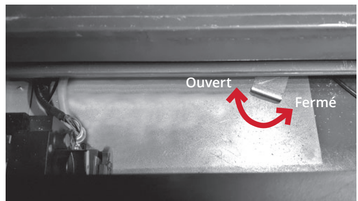
Vu du haut—Levier d'ajustement de l'obturateur d'air situé sous la boîte de foyer derrière le panneau avant de l'appareil
