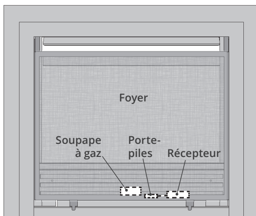
Porte-piles situé à côté du récepteur sous la boîte de foyer derrière le panneau d'accès.
