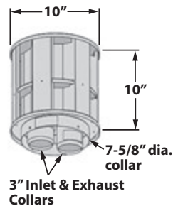
Sortie colinéaire typique
