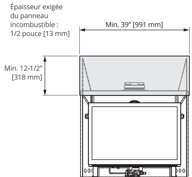
Dimensions minimales du panneau de béton
