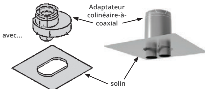
Sortie coaxiale
